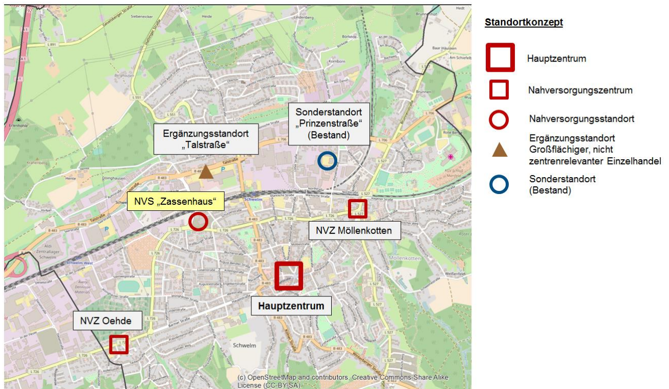
Karte 17: Fortgeschriebenes Standortkonzept für den Einzelhandel 2017
